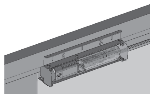
AUTOMATIZADOR RAC SEM O ACABAMENTO
