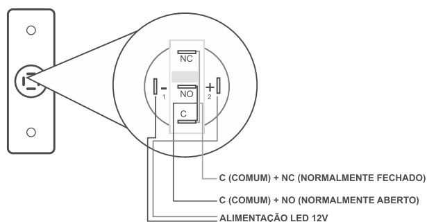
ESQUEMA DE LIGAÇÃO
